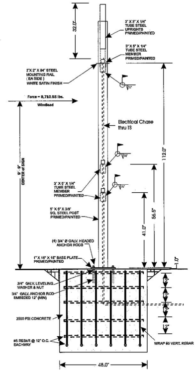
SECTION Scale: 3/8" = 1'-0"
